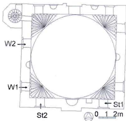
Rys. 3. Plan budowli i lokalizacje, z których pobrano kamienie
