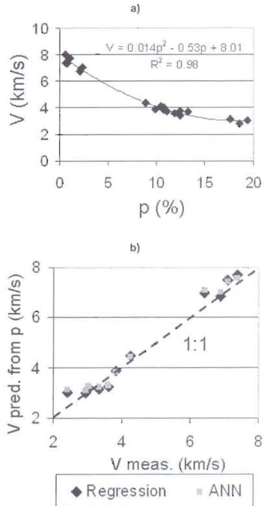
Rys. 12 (a) Model regresji zależności V-p (b) V estymowane z wartości p w zależności od mierzonego V
