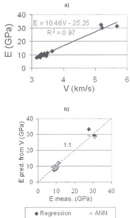
Rys. 8 (a) Model regresji zależności E - V (b) E prognozowane z wartości V w zależności od mierzonego E
