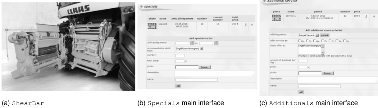
Fig. 6. SUCs.
