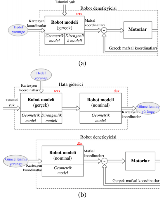
Şekil 3. Direngenlik modeli eklenmiş denetim algoritmaları: Direngenlik modelinin (a) Çevrimiçi kullanımı, (b) Çevrimdışı kullanımı [34]
