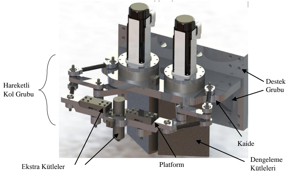
Şekil 4. Konstrüksiyonel tasarım
