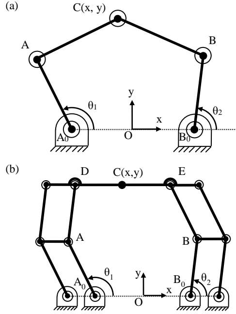
Şekil 1. a) Normal kısıtlı 5R mekanizması, (b) Fazla kısıtlı 6R mekanizması
