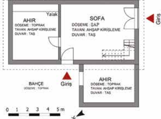
Şek. 10: Zemin kat planı Fig. 10: Ground-floor plan
